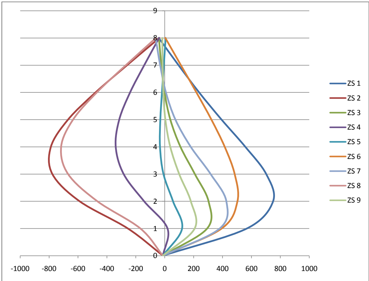
Porovnanie obvodových ťahov N_x [kN/m]
