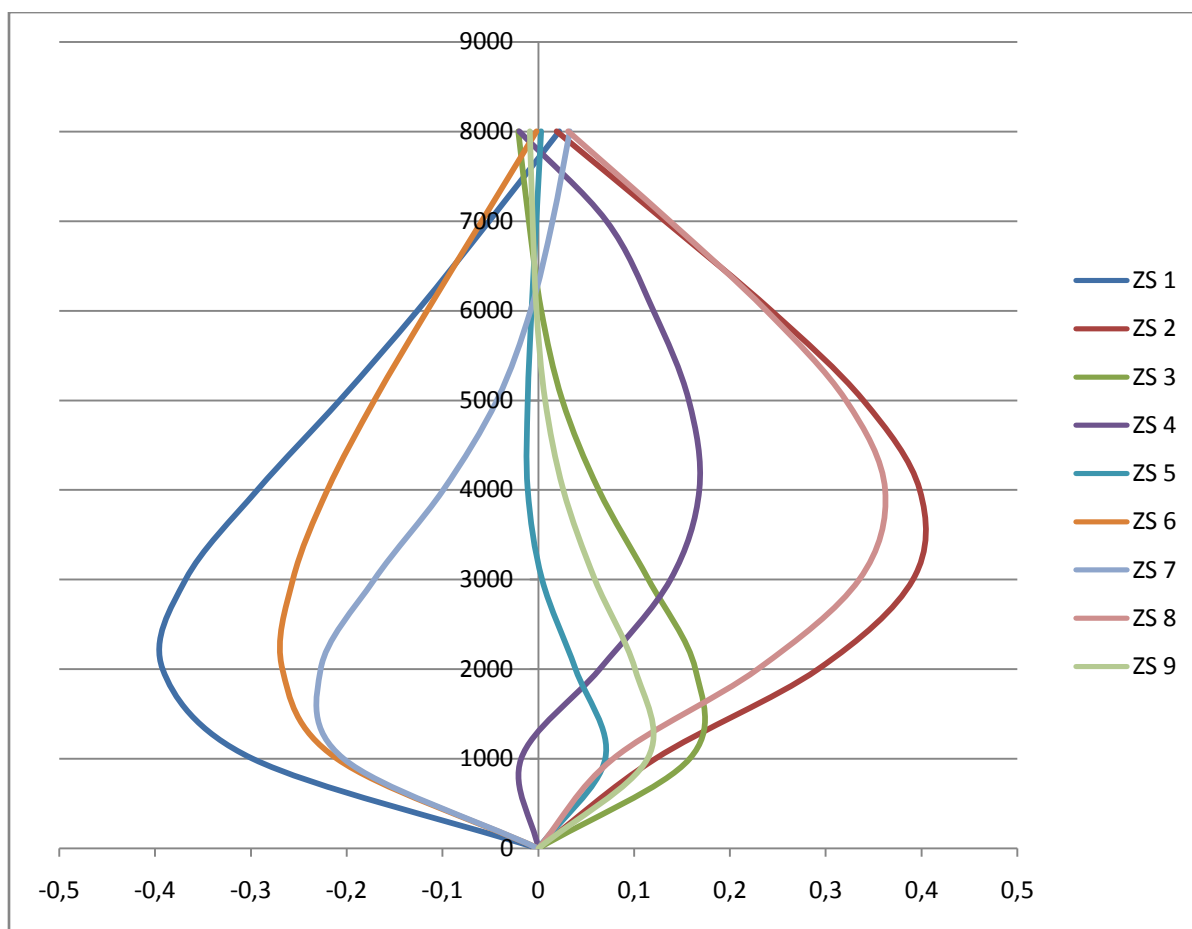
Porovnanie deformácií ux [mm]
