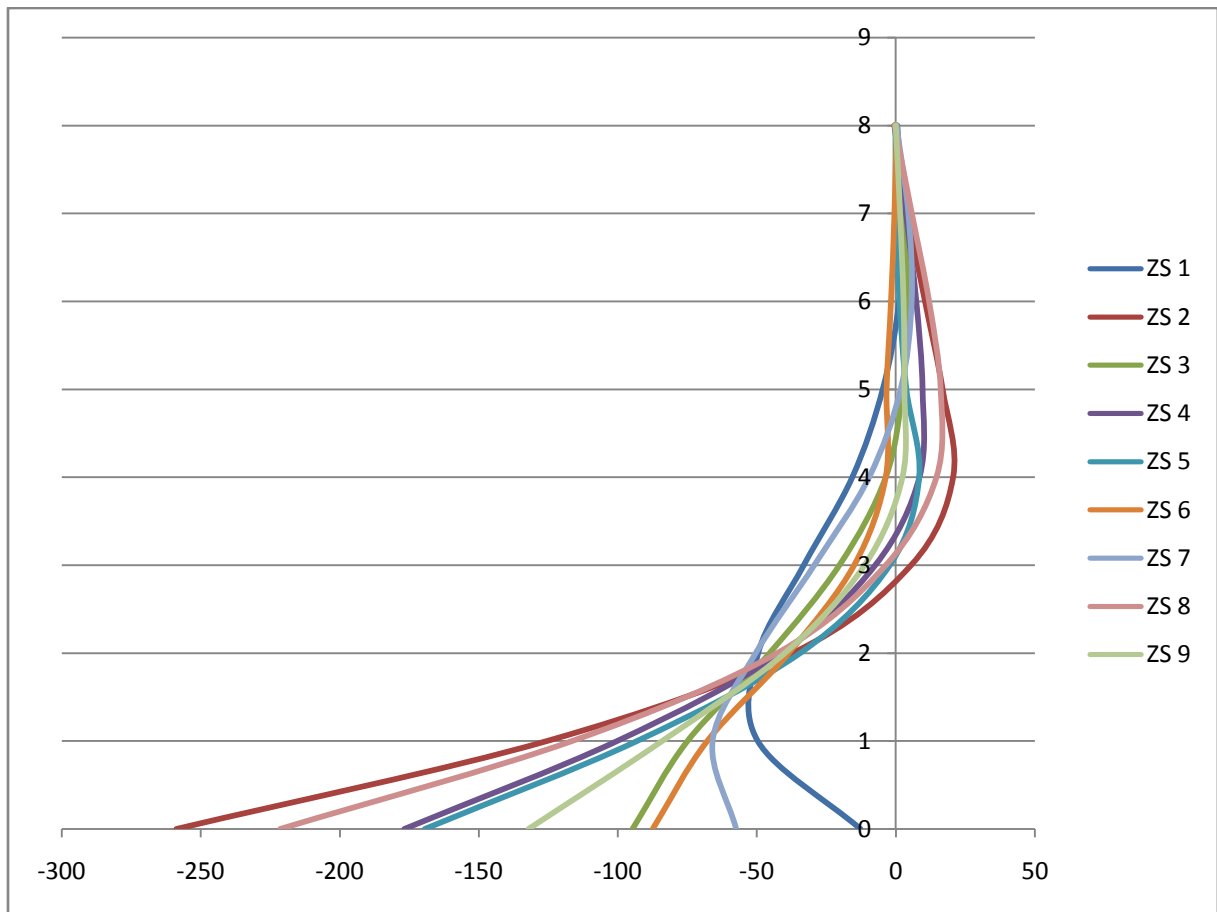
Porovnanie priečnych síl V_x [kN/m]
