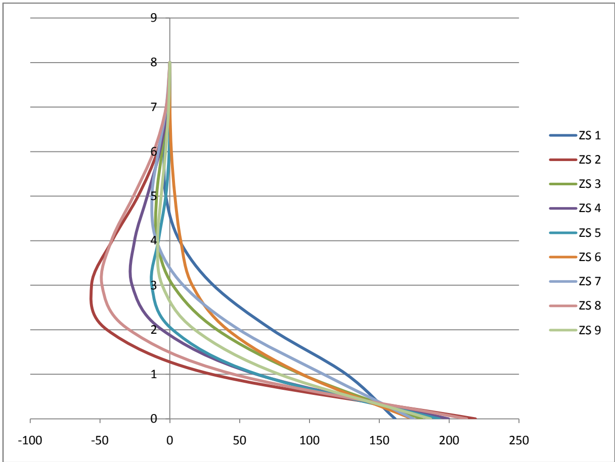
Porovnanie ohybových momentov M_x [kNm/m]
