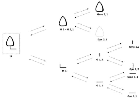
Obr. 55: Schéma morfografickej analýzy objektu „orientačný strom“ (3VM)
