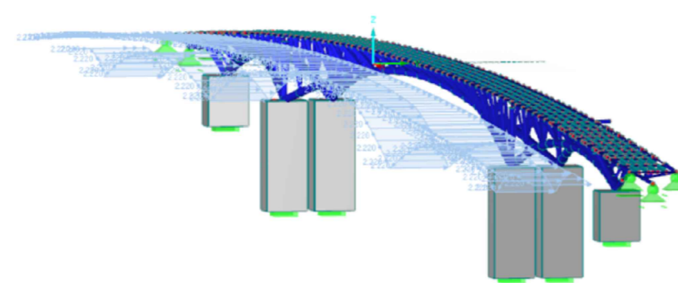
Schéma zaťaženia vetrom pre 1. variant
