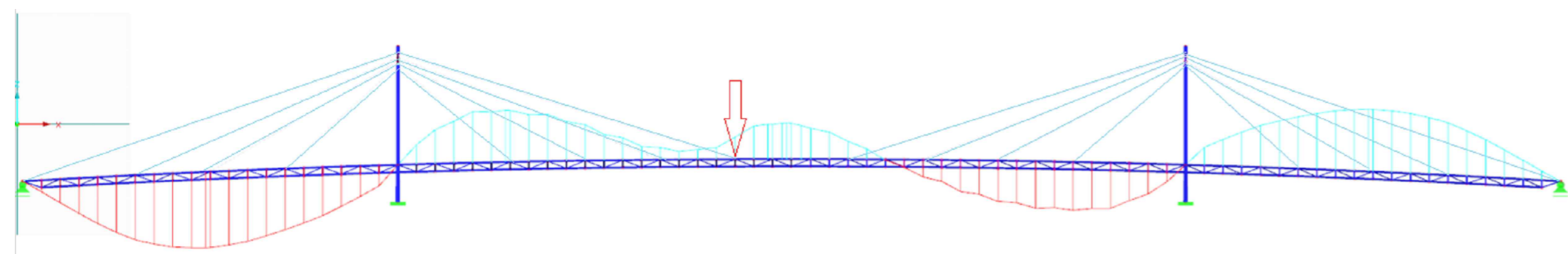
Vplyvová čiara pre horné lano
