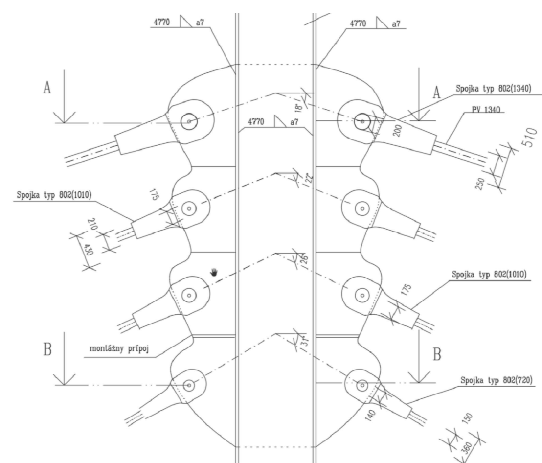
Detail ukotvenie lán k pylónu
