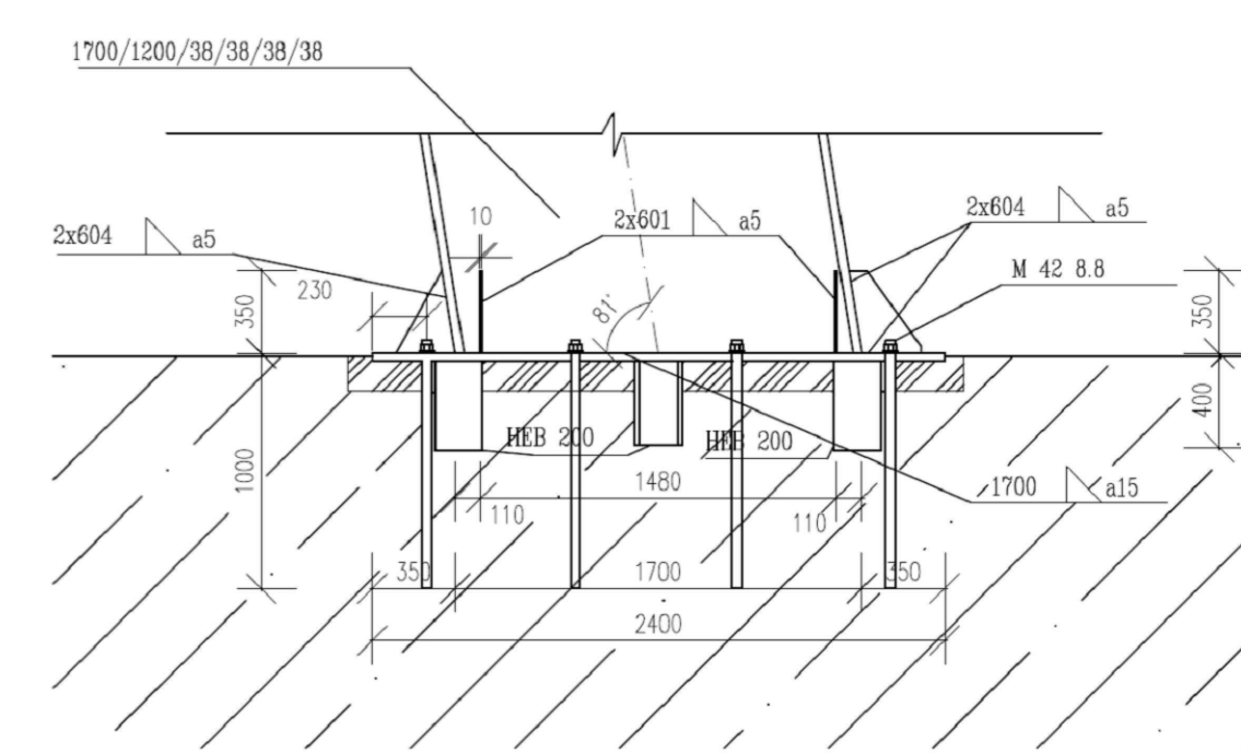
Detail ukotvenia pylóna
