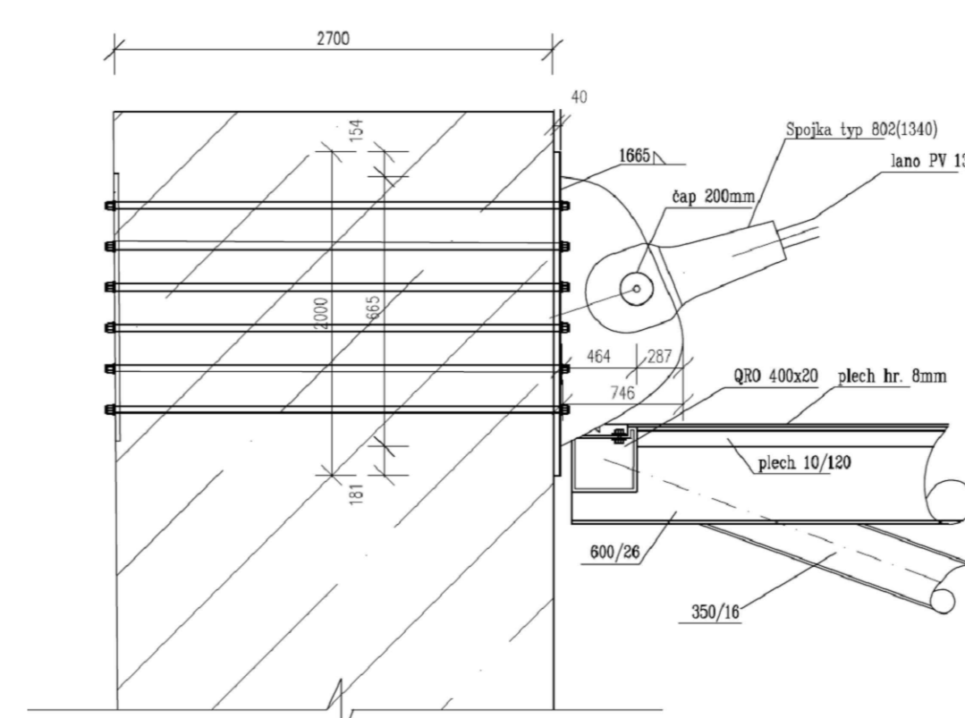
Detail ukotvenia lana k základu a uloženia na posúvne závery
