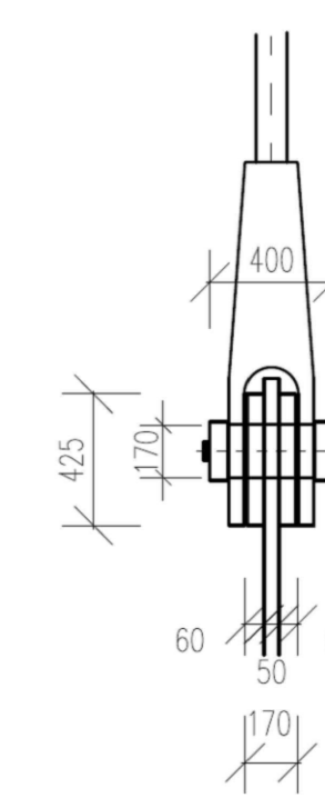
Detail spojky lana
