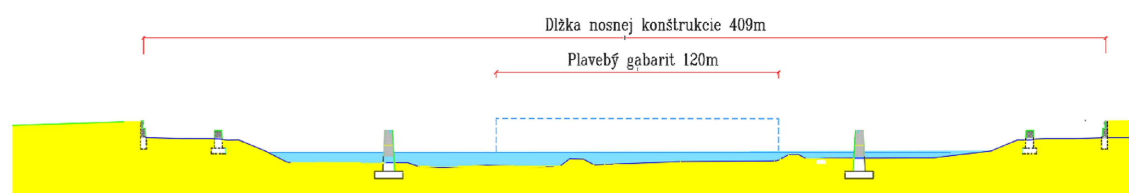
Schéma plavebného gabaritu a dĺžky konštrukcie
