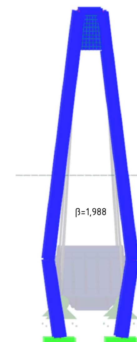
Schéma pre výpočet stability rámu
