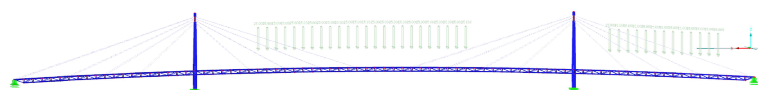
Zaťažovací stav vygenerovaný na základe vplyvovej čiary
