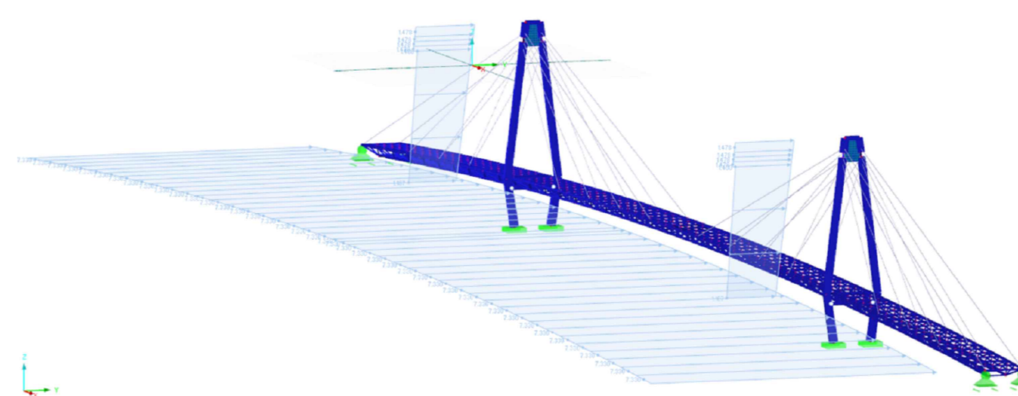
Schéma zaťaženia vetrom pre 2. a 3. variant
