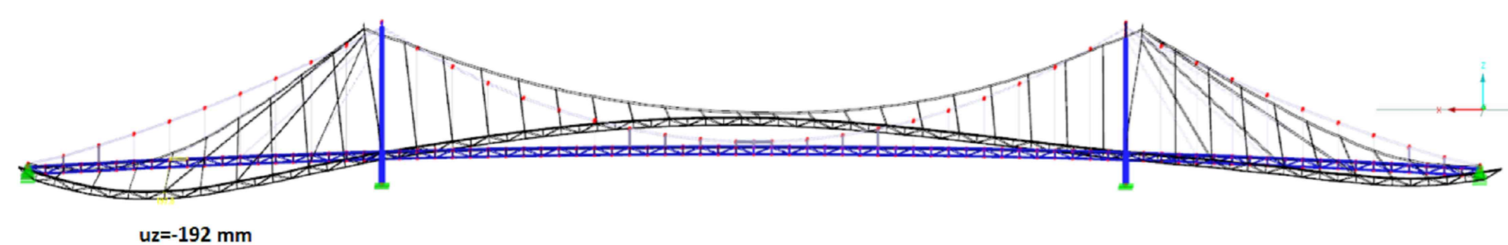
2. variant - častá kombinácia
